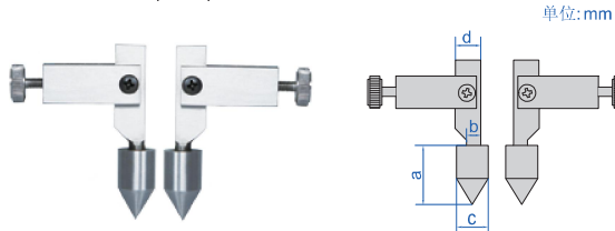
中心距测头(选配)
