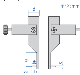
圆柱沟槽测头(选配)
