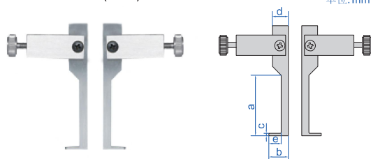
扁头沟槽测头(选配)
